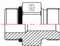
MORB-MBSPP Straight
