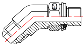
MJ-MBSPP ADJ. 45° Elbow
