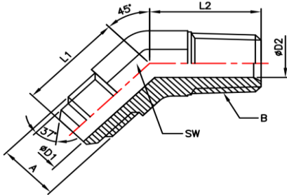
MJ-MBSPP 45° Elbow
