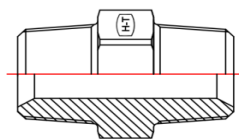
MBSPT-MBSPT Straight
